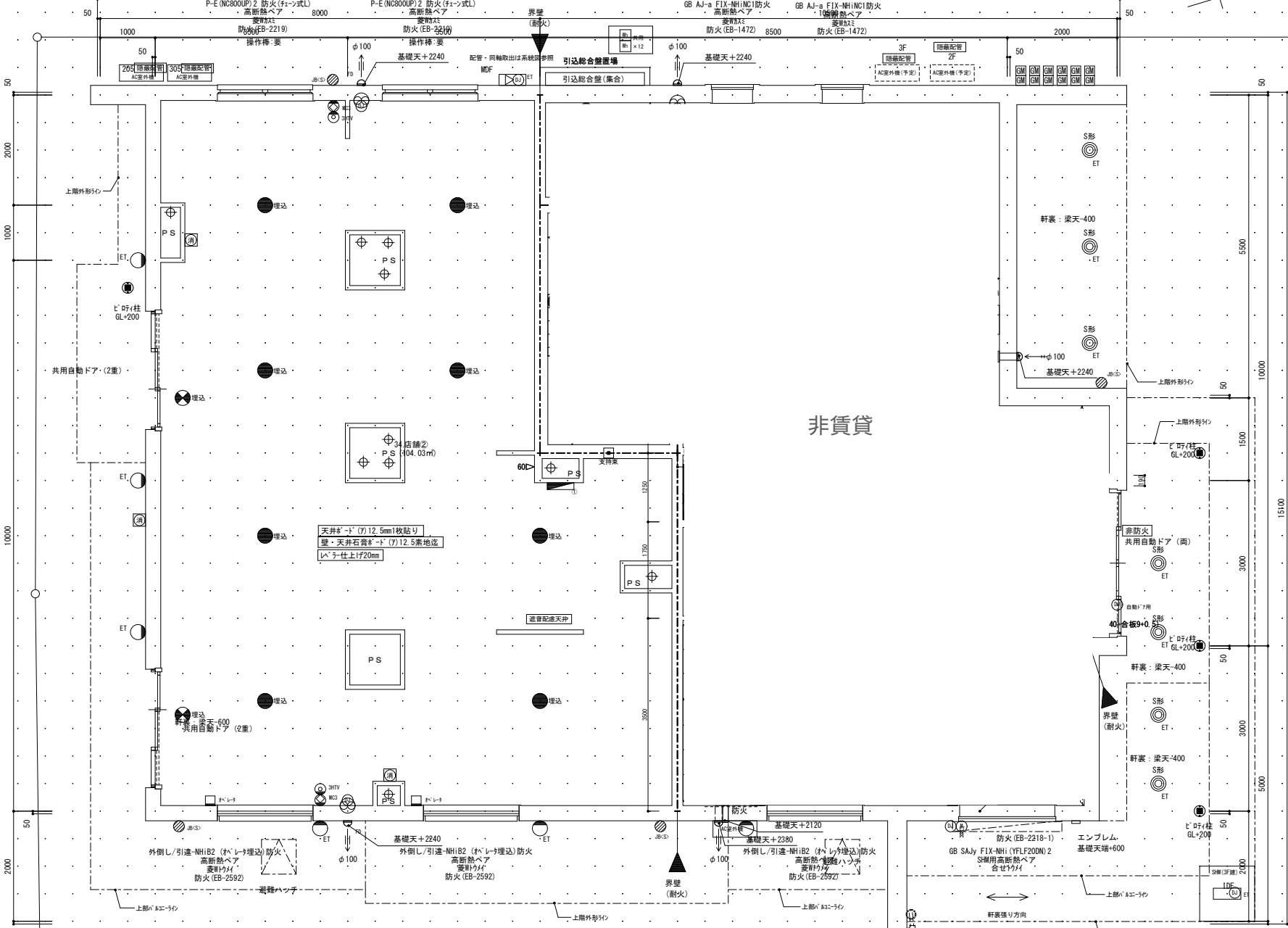
1階平面図 1/50
